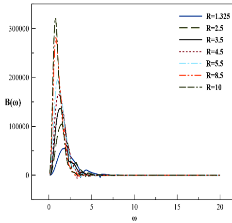
Figure 10 : Amortissement hydrodynamique B(\omega) en fonction de \omega .
