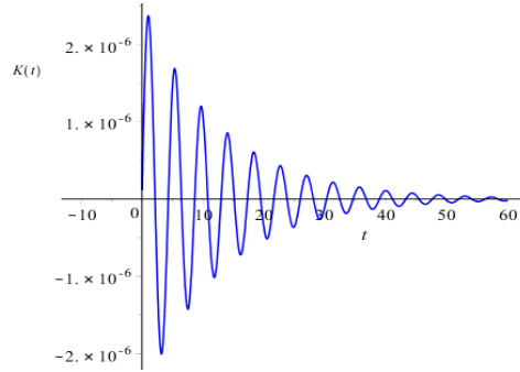
Figure 16 : Fonction de réponse impulsionnelle K_{ii}(t) dans le cas où V_m = 30 m.s^{-1} .
