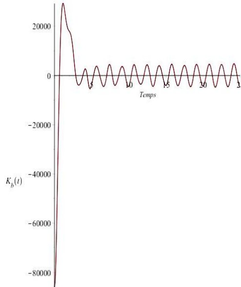
Figure 7 : Fonction de réponse impulsionnelle K_b(t) .
