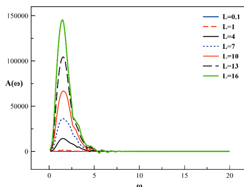
Figure 12 : Masse ajoutée A(\omega) en fonction de \omega .
