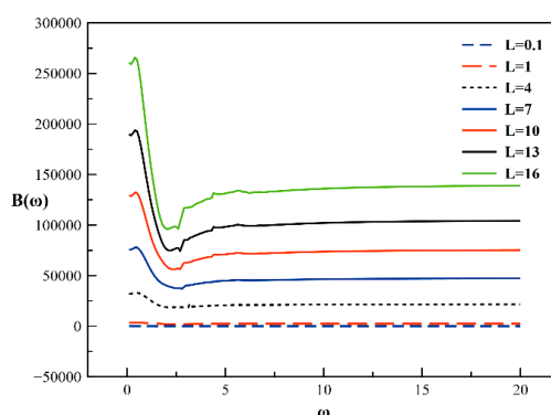
Figure 13 : Amortissement hydrodynamique B(\omega) en fonction de \omega .
