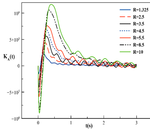
Figure 11 : Fonction de réponse impulsionnelle K_a(t) .
