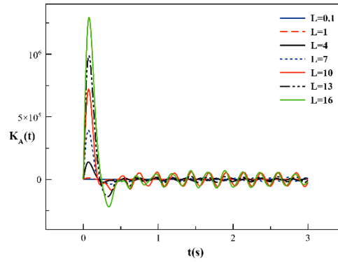
Figure 14 : Fonction de réponse impulsionnelle K_a(t) .
