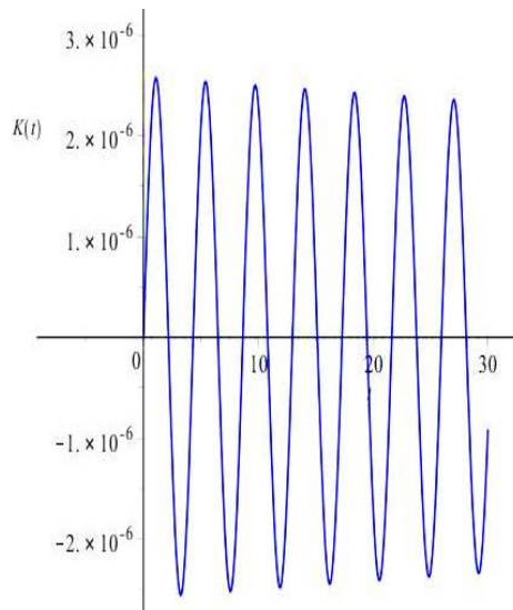
Figure 15 : Fonction de réponse impulsionnelle K_{ii}(t) dans le cas où V_m = 1.3 \text{ m.s}^{-1} .
