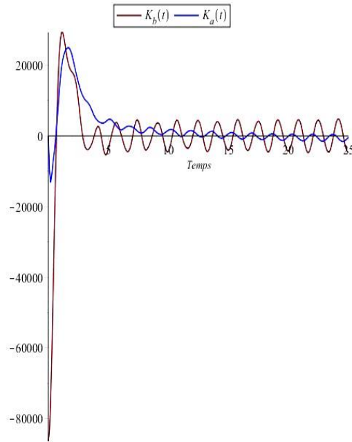
Figure 8 : Comparaison entre la réponse impulsionnelle K_a(t) et K_b(t) .
