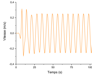
Figure 4 : Vitesse v(t) en fonction de t .
