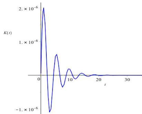
Figure 17 : Fonction de réponse impulsionnelle K_{ii}(t) dans le cas où V_m = 100 m.s^{-1} .
