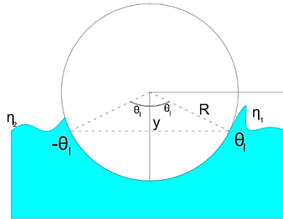
Figure 2 : Schéma en 2D du cylindre flottant.
