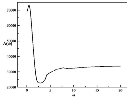
Figure 5 : Masse ajoutée A(\omega) en fonction de \omega .
